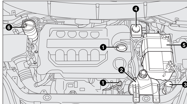
şekil 203 – 1.6 Multijet tipleri
