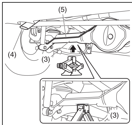
後輪
