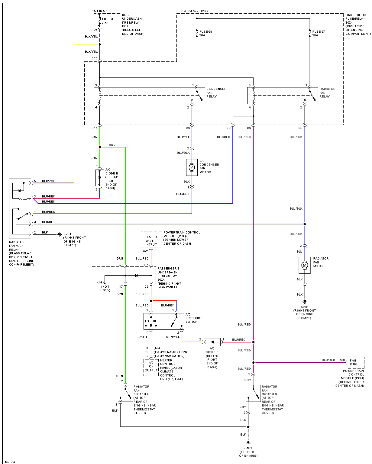
Fig. 19: Cooling Fan Circuit
