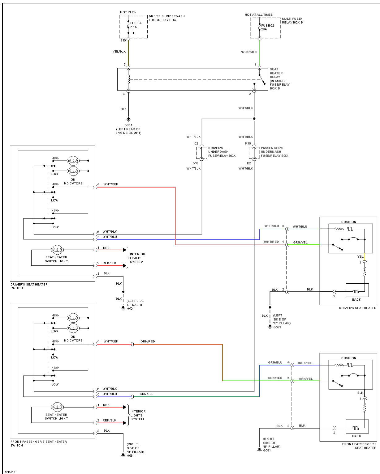
Fig. 60: Heater Circuit
