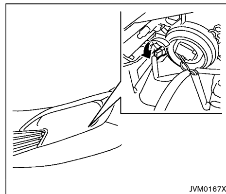
車幅灯
