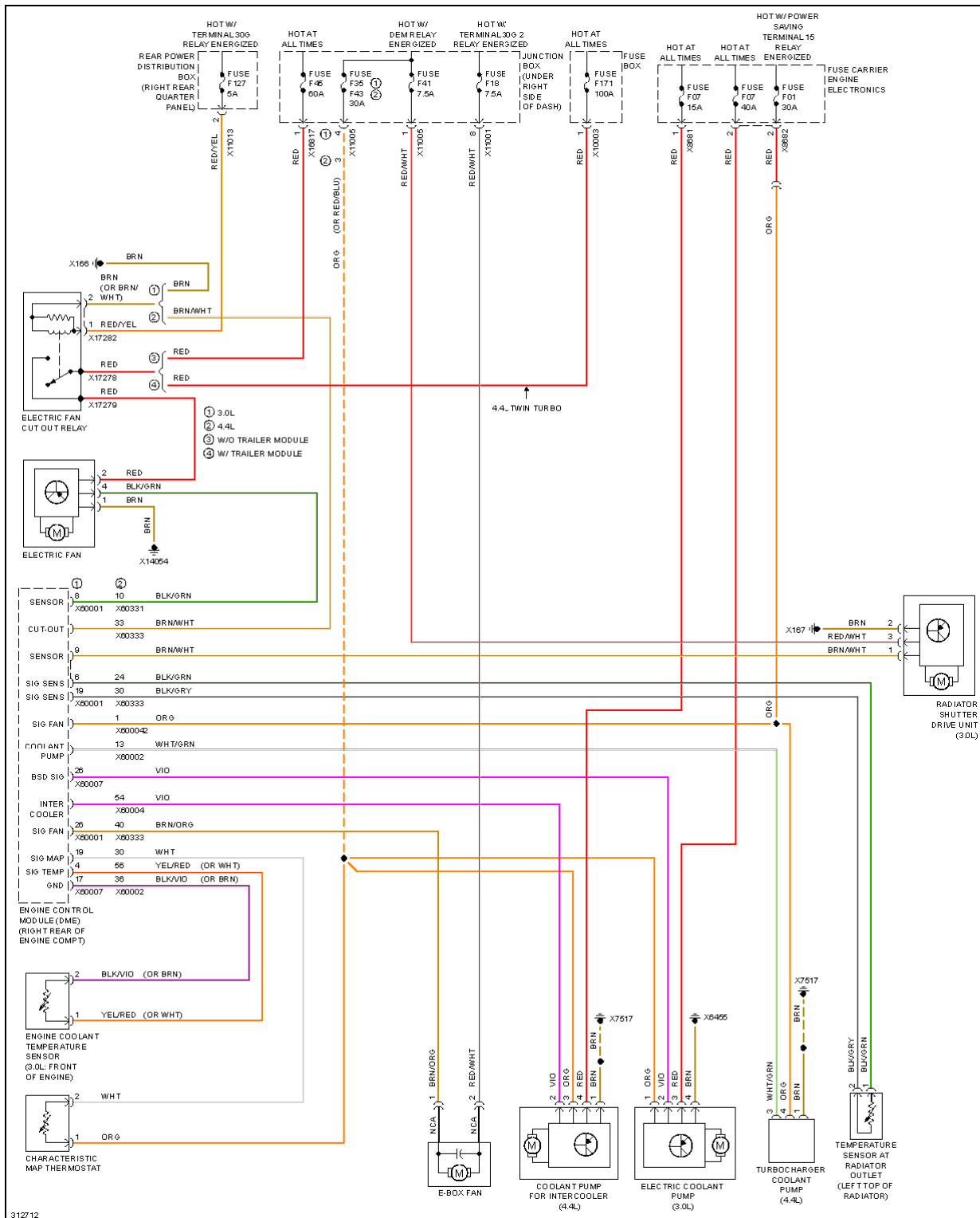
Fig. 21: Cooling Fan Circuit
