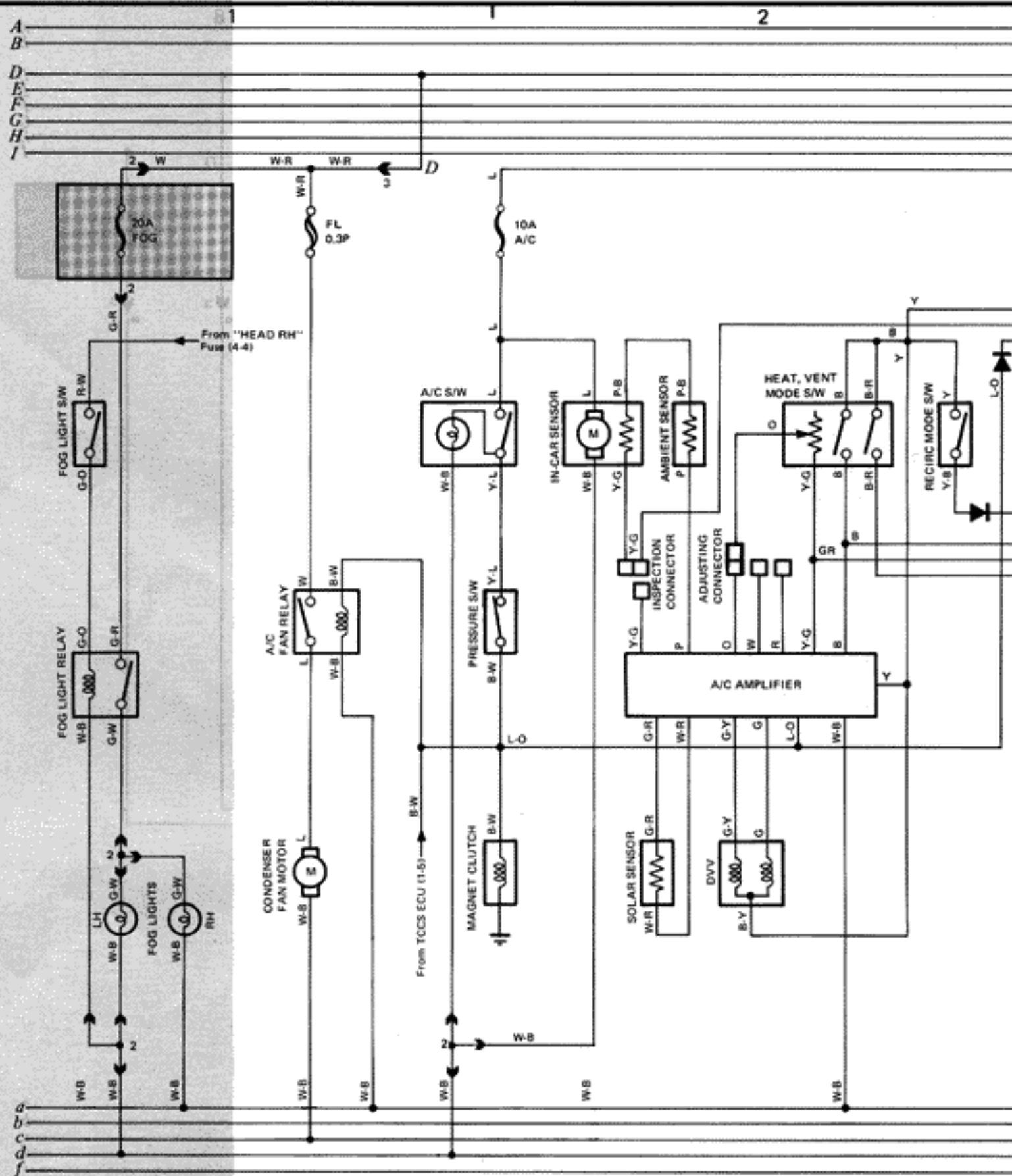
Fog Lights
