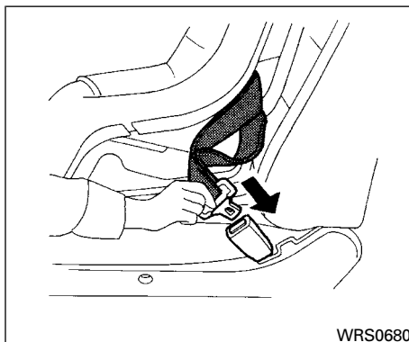
Orientación hacia adelante – paso 3
