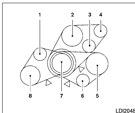
Modelo YD25DDTi
