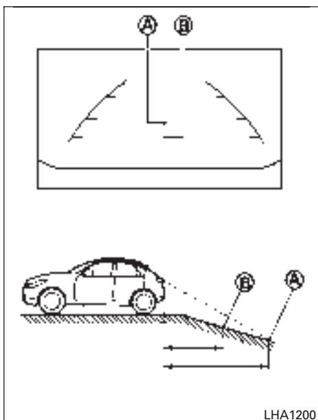
Movimiento de reversa en una pendiente descendente pronunciada
