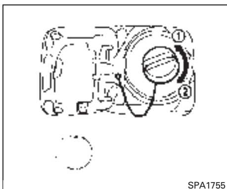
Tanque trasero TAPÓN DE LLENADO DE COMBUSTIBLE (vehículos con combustible flexible, solo Brasil)
