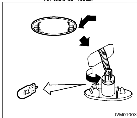
方向指示器（側面）
