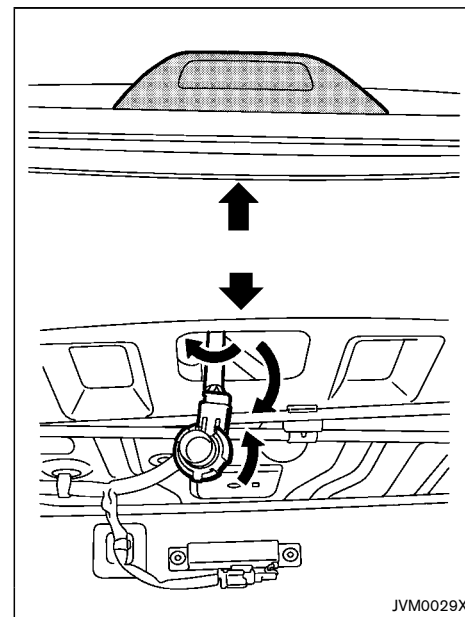
ハイマウントストップランプ
