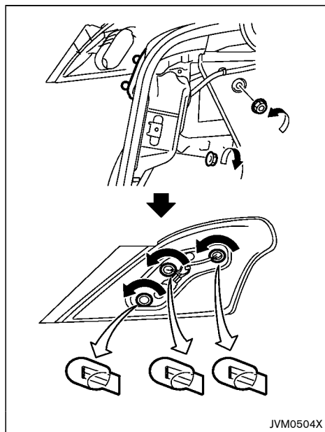
リヤコンビランプ
