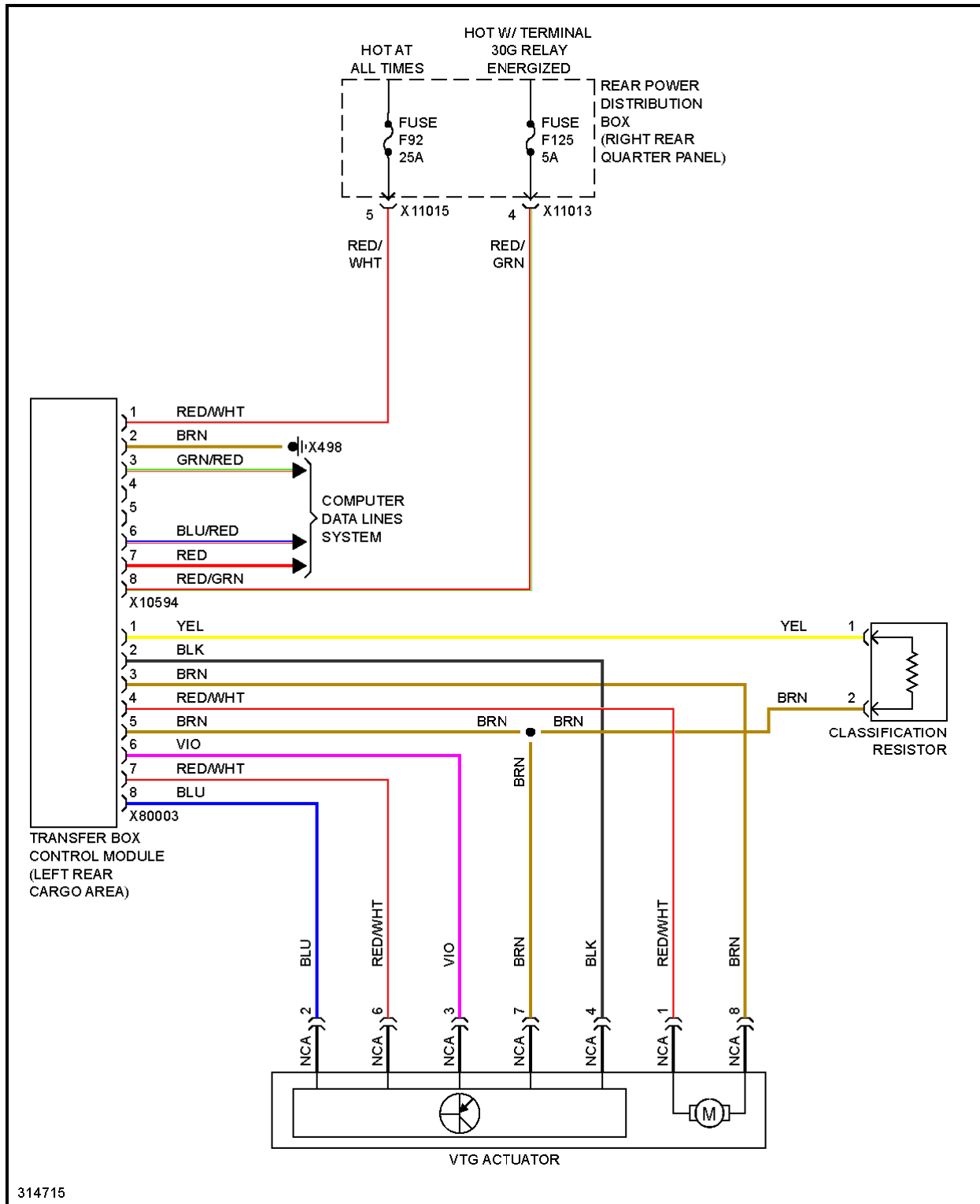
Fig. 123: AWD Circuit
