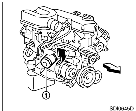
Motor KA24DE
