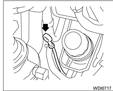
Motor YD25DDTi
