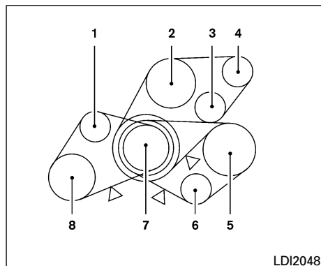
Modelo YD25DDTi
