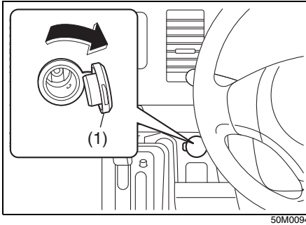
(1) ふた
