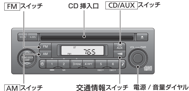
AM/FM チューナー付き CD プレーヤー
