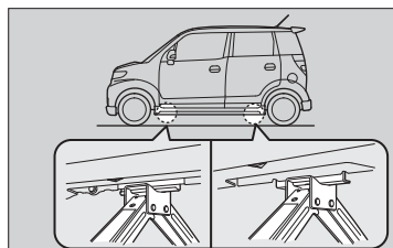
サイドスポイラー装備車
