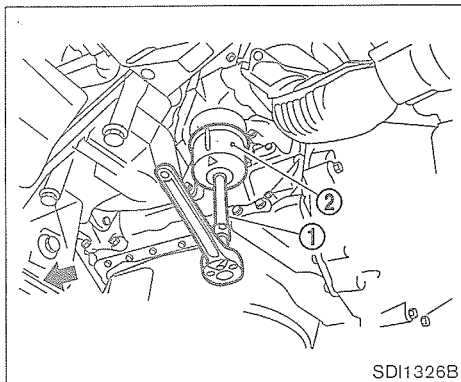
Motor ZD30DD/DDTi
