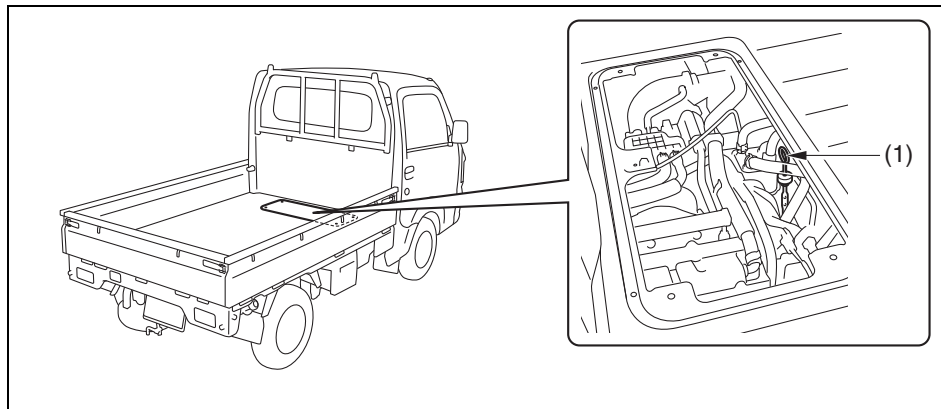
(1) トランスミッションフルードレベルゲージ(AT車)
