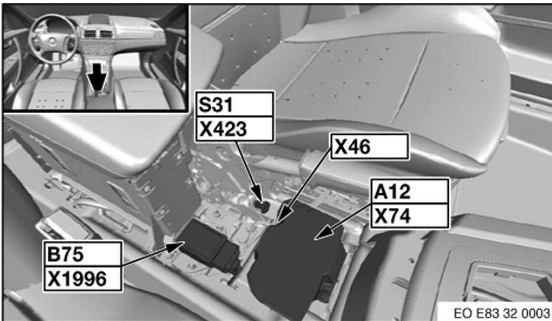
Fig. 19: Center Console
