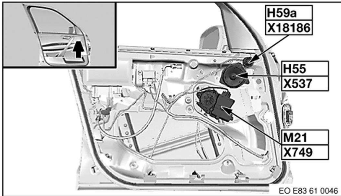
Fig. 61: Driver's Door
