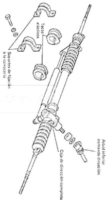
Fig. 6.11 y 6.12 Particulares componentes la caja de direccion con amortiguador
