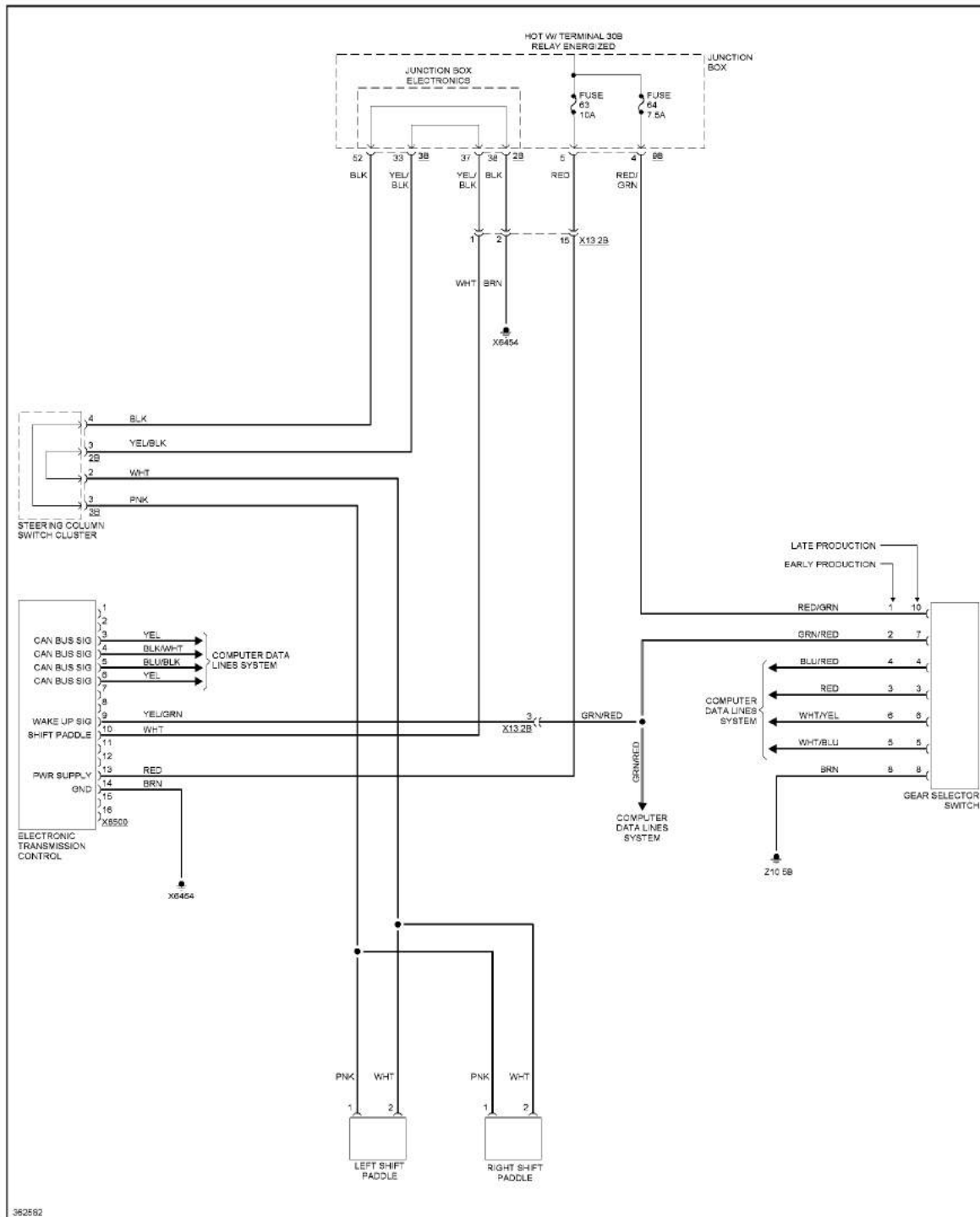
Fig. 89: A/T Circuit
