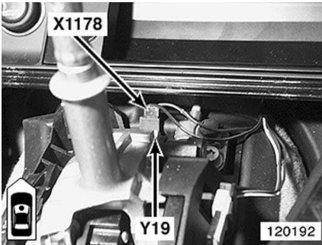
Fig. 59: Center Console
