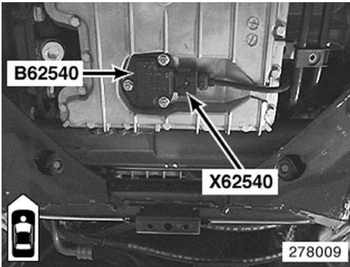
Fig. 37: Oil Pan
