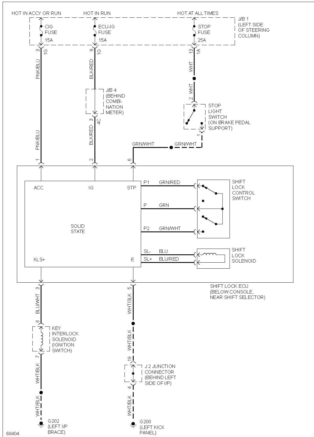
Fig. 54: Shift Interlock Circuit
