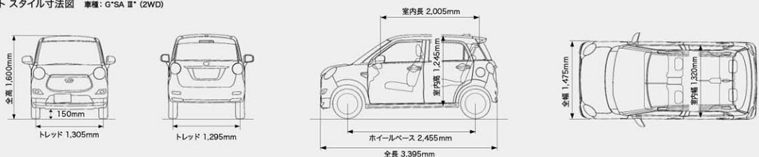
キャスト スタイル寸法図 車種: G"SA III" (2WD)
