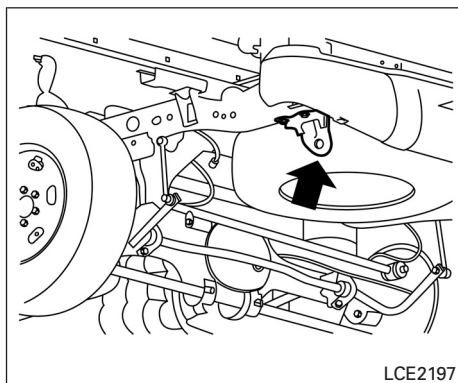
Gancho de recuperación trasero tipo A (solo si está equipado)
