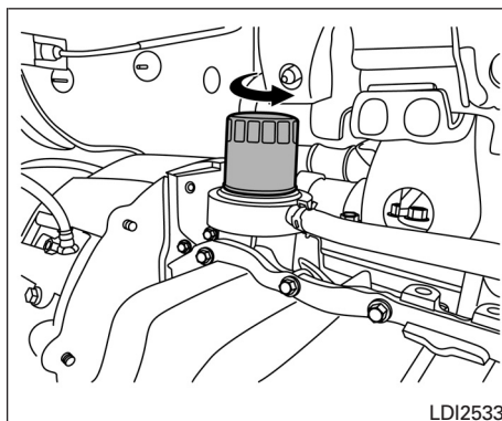
Motor QR25DE
