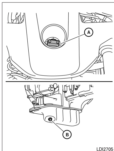
Motor YD25DDTi
