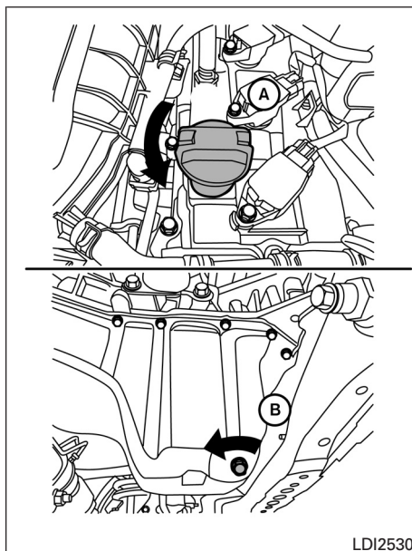
Motor QR25DE
