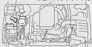
メインヒューズ ヒューズボックスNo. 1
