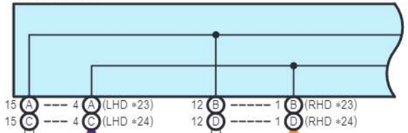
E75(A), E87(B), E111(C), E112(D) Junction Connector
