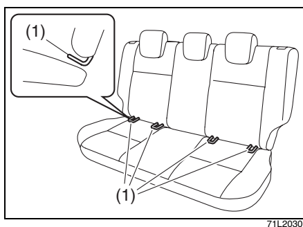
(1) ISOFIXアンカー
