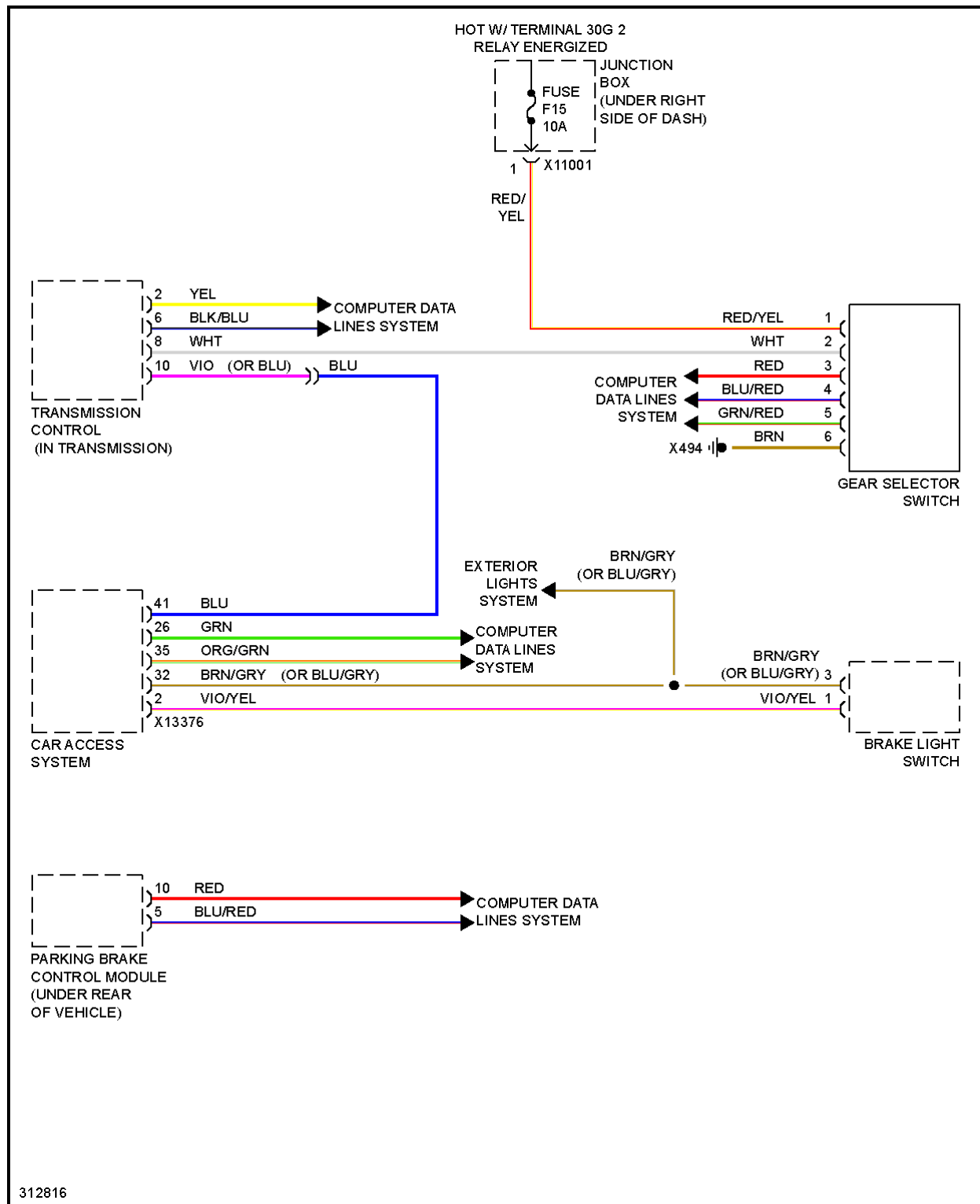
Fig. 117: Shift Interlock Circuit
