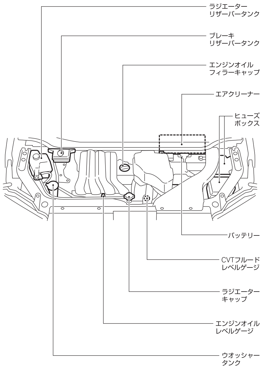
■エンジンルーム内配置図
