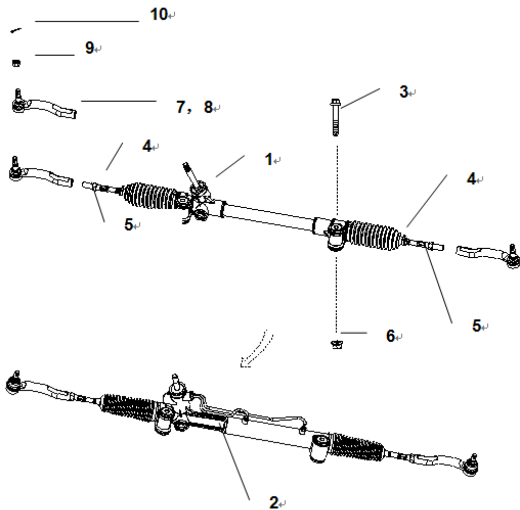
图 2.11.4 转向泵总成
