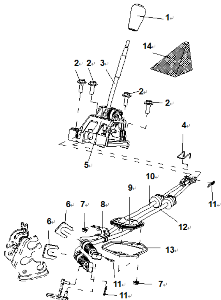
图 2.6.3 换档操纵机构总成 (AMT)
