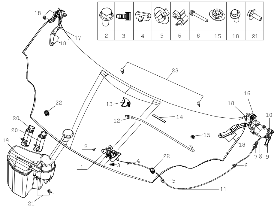
图 4. 1. 1 发动机罩附件
