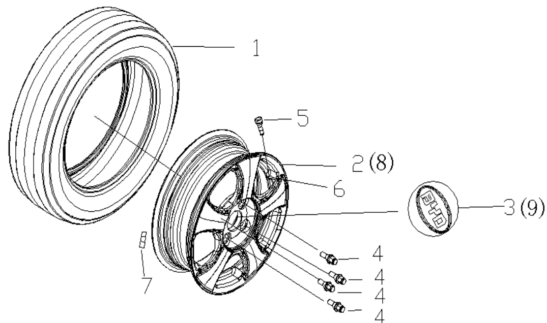
图 2.12.2 铝轮-轮胎（豪华型、尊贵型）
