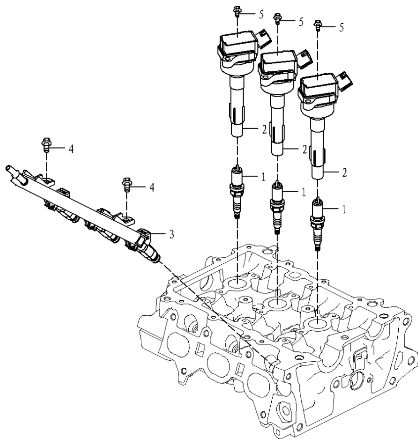
图 1. 1. 18 发动机传感器
