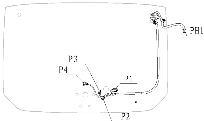
图 3.2.6 后背门左线束
