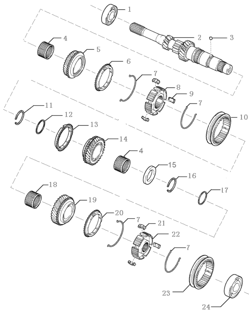
图 1.2.5 副轴组件
