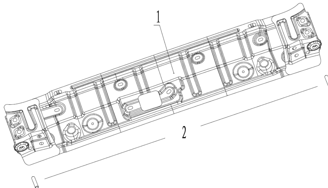
图 6.18 顶盖后横梁总成
