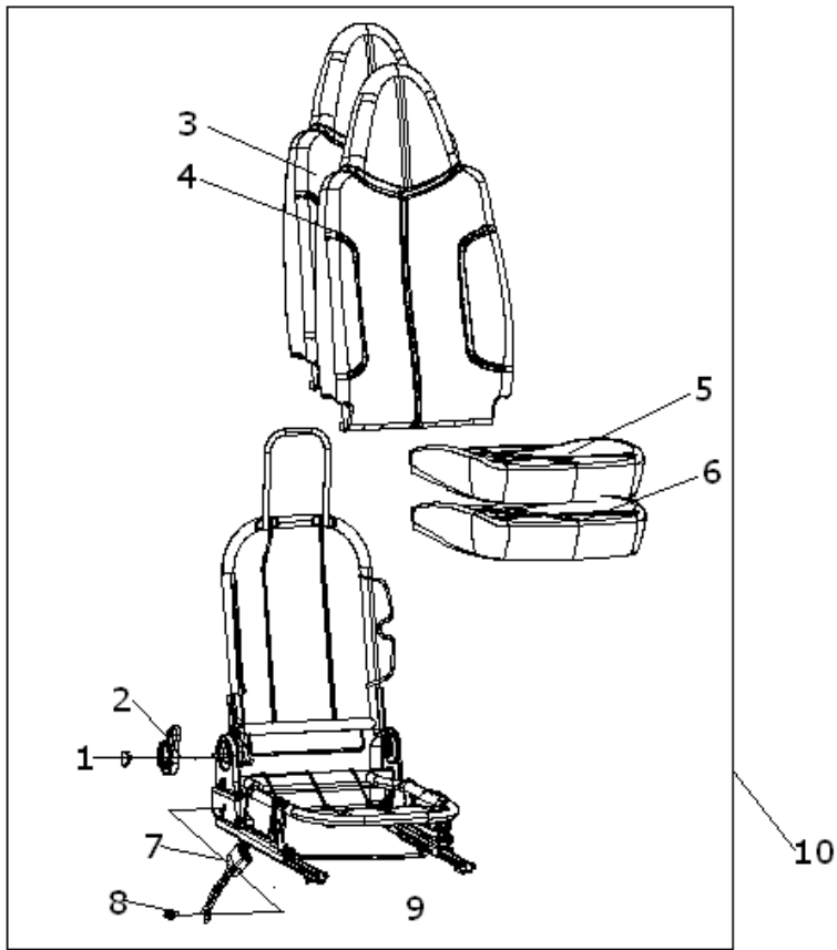
图 4. 1. 13 副驾驶座椅总成
