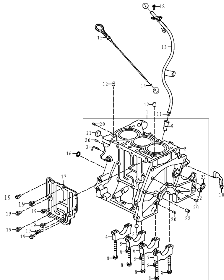
图 1. 1. 1-3 气缸体组件
