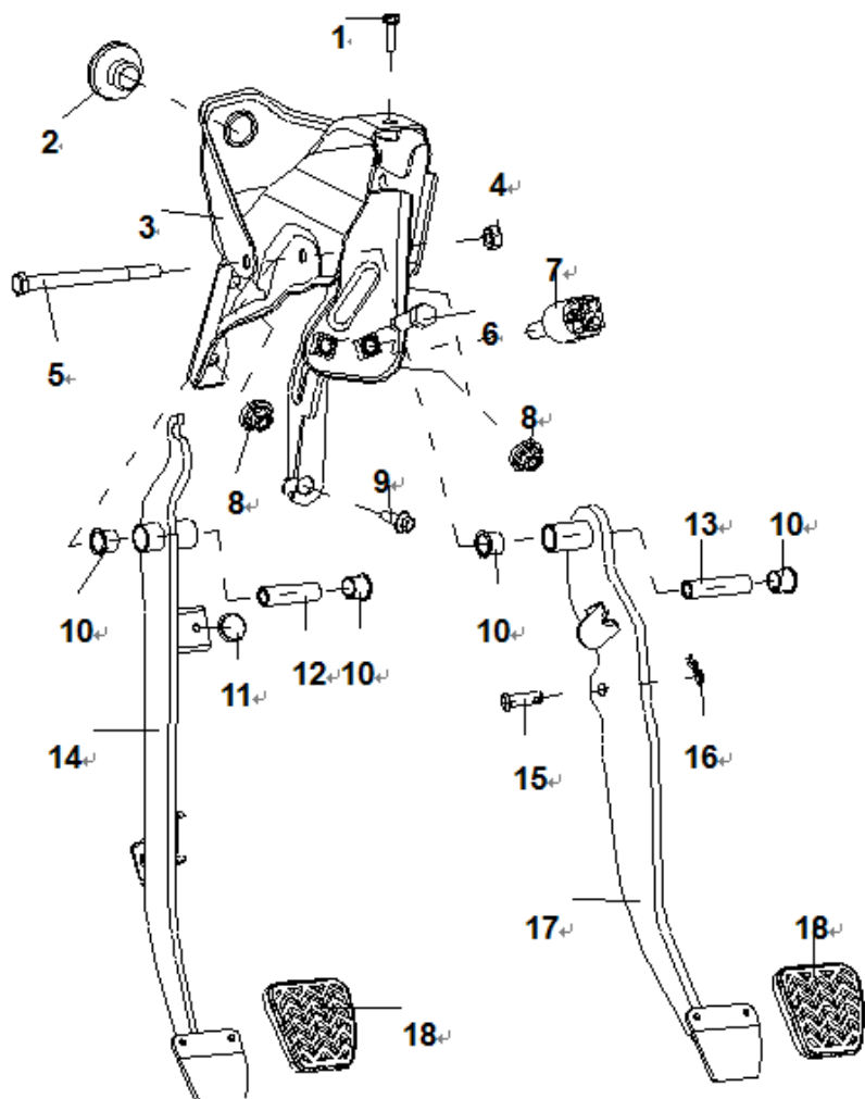
图 2.6.1 制动离合踏板及支架总成
