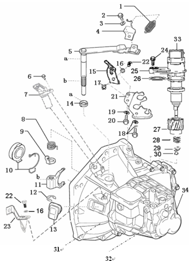
图 1.2.1 变速箱外部零部件
