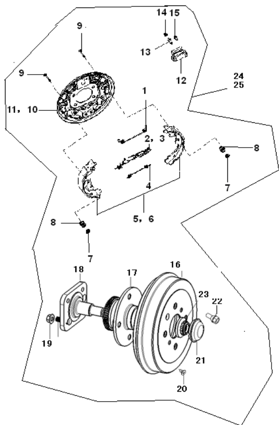
图 2.4.2-1 后制动器总成
