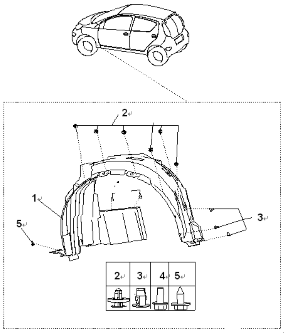
图 5.1.7 左前轮罩挡泥板
