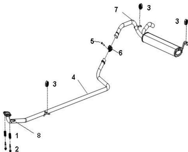
图 2.2.1 排气系统
