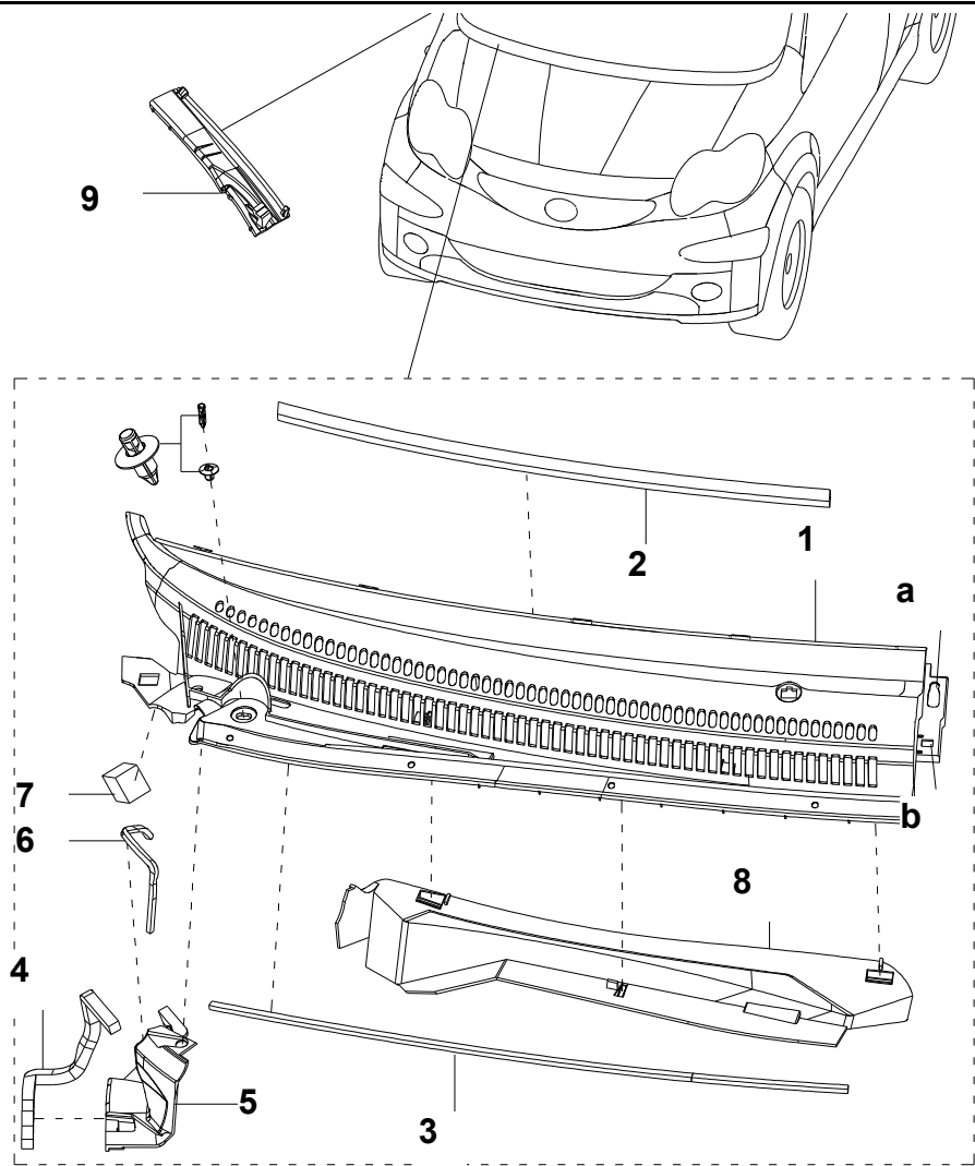
图 5.1.5 翼子板角饰板 、车轮装饰罩和后通风口总成
