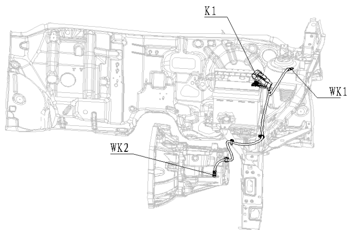
图 3.2.7 负极线束
