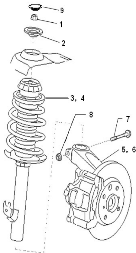
图 2.8.2 前减振器总成
