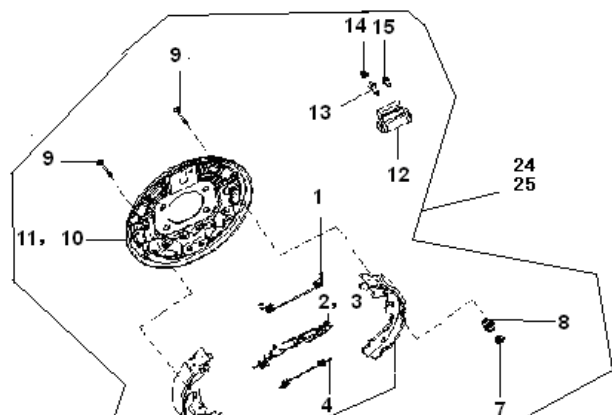
图 2.4.2-1 后制动器总成
