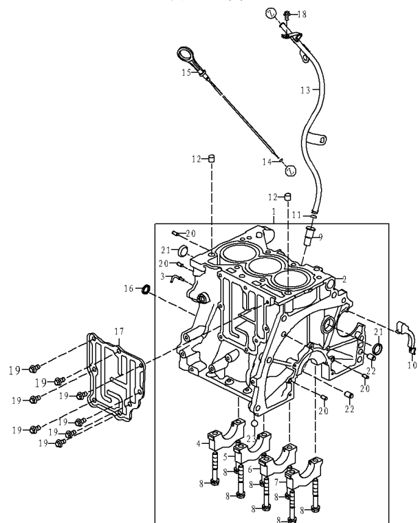
图 1.1.1-3 气缸体组件
