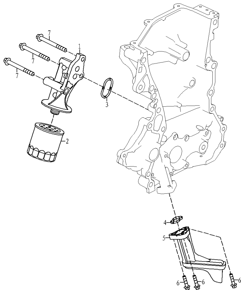
图 1. 1. 9 正时罩及附件
