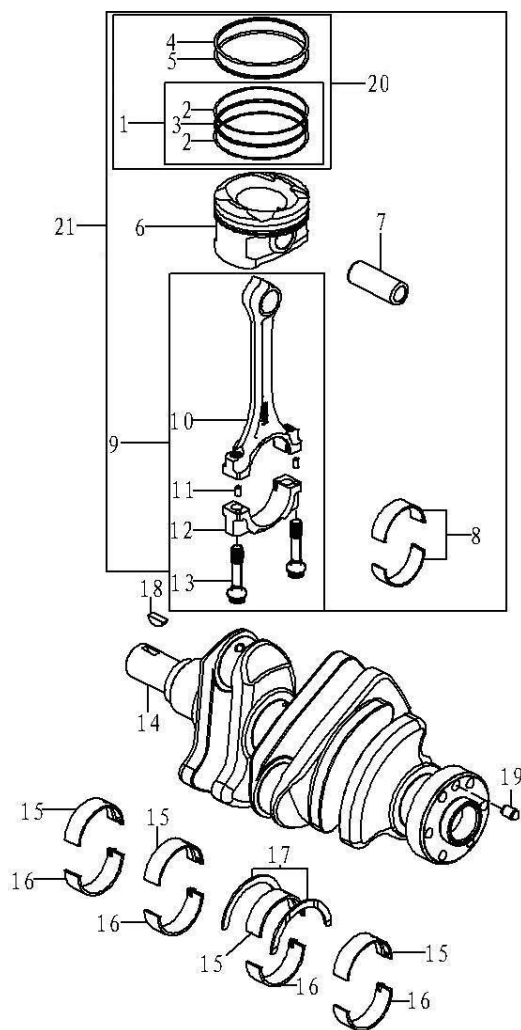
图 1. 1. 3 曲轴活塞连杆机构
