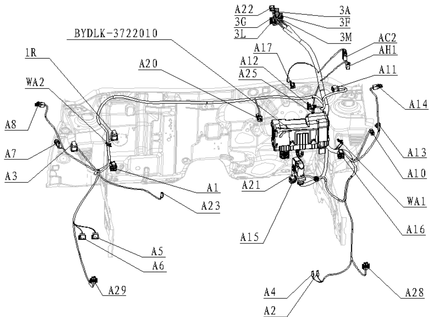
图 3.2.10 前舱线束
