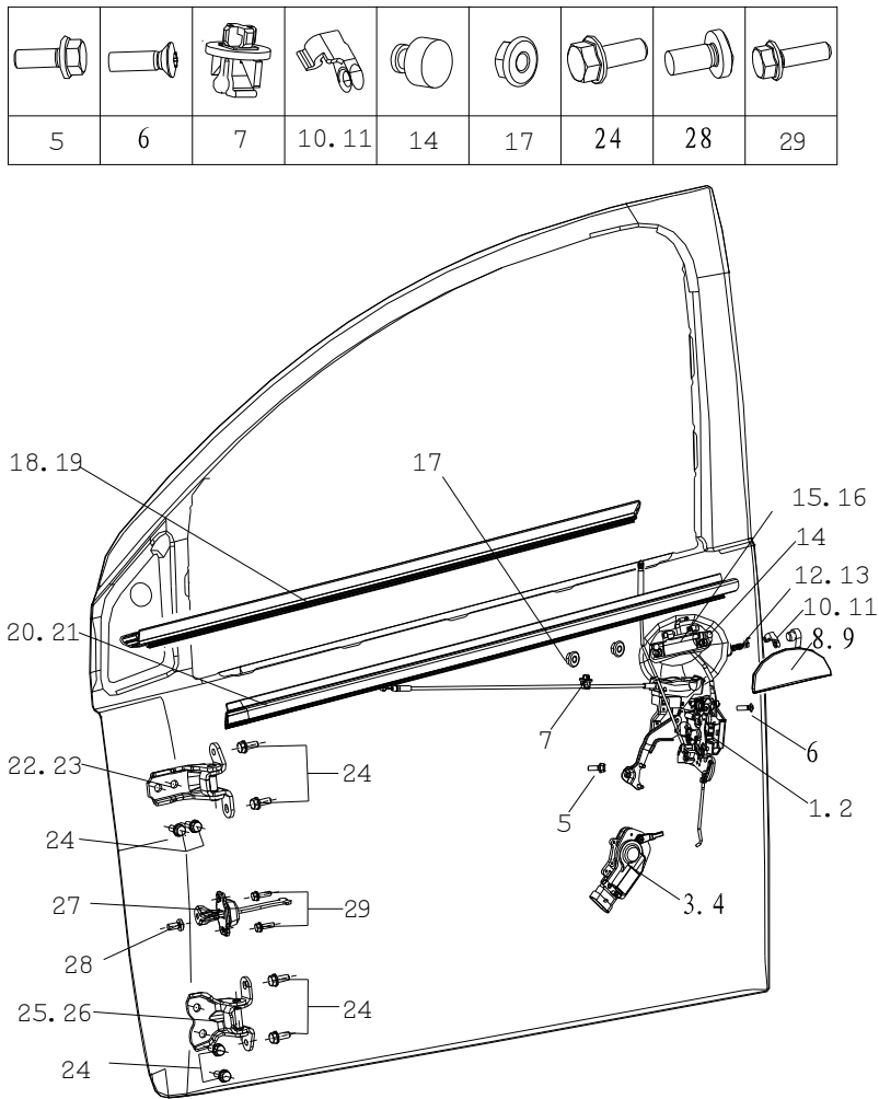
图 4. 1. 4 前门玻璃升降器
