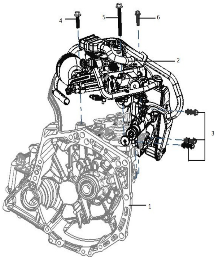
图 1.3.2 变速器外部零部件
