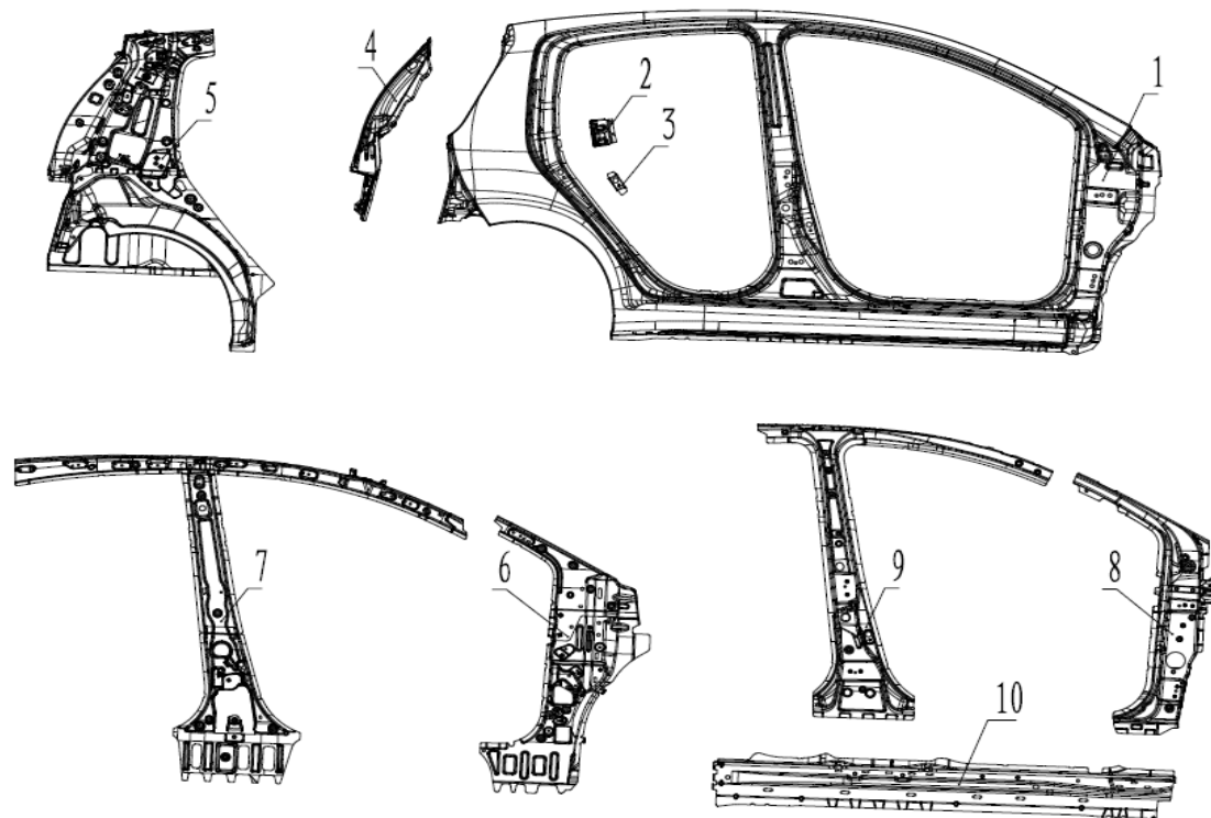
图 6.15 右侧围总成
