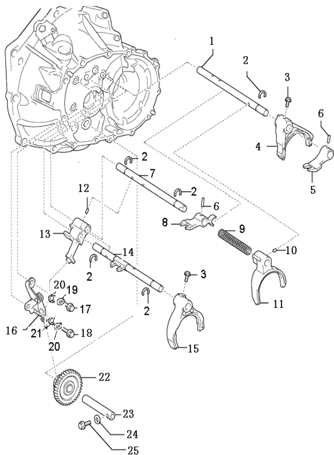
图 1.3.5 换挡杆及换挡拨叉
