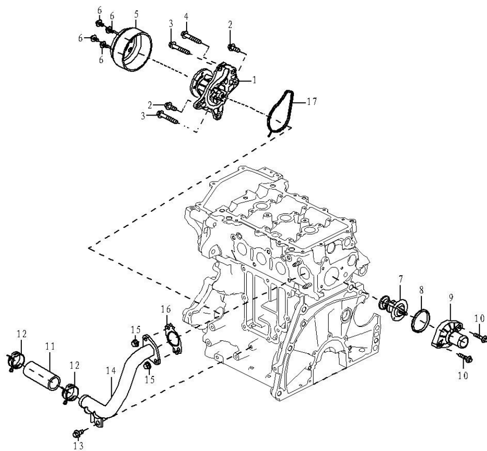
图 1.1.13 冷却系统
