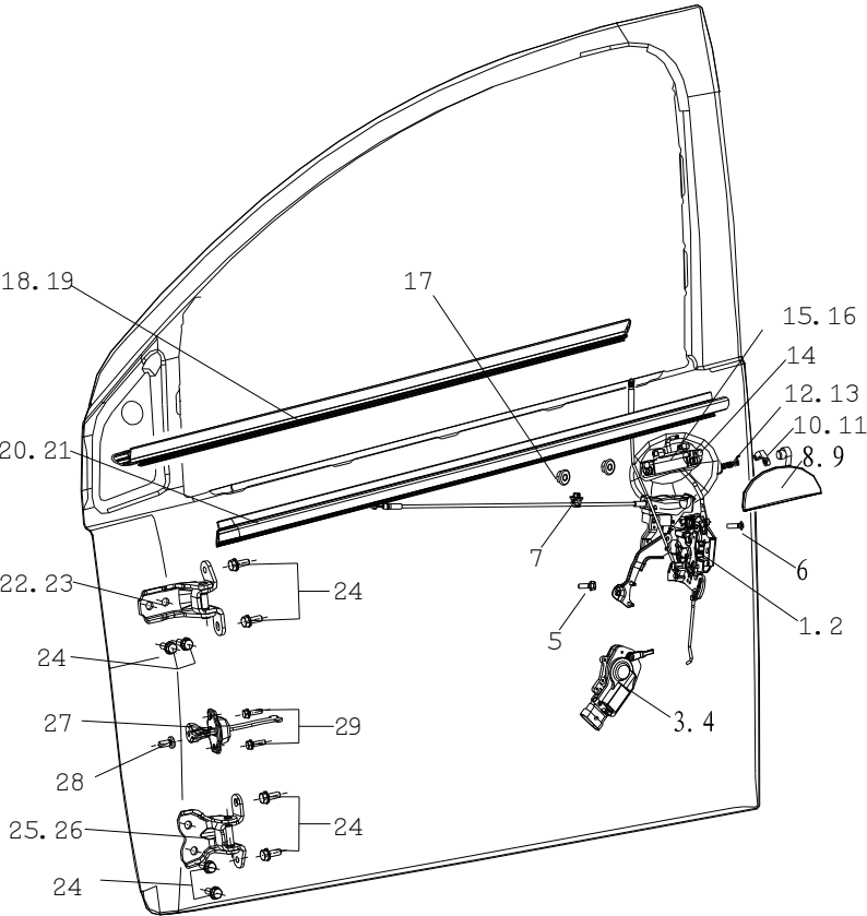
图 4. 1. 3 前门锁及前门铰链
