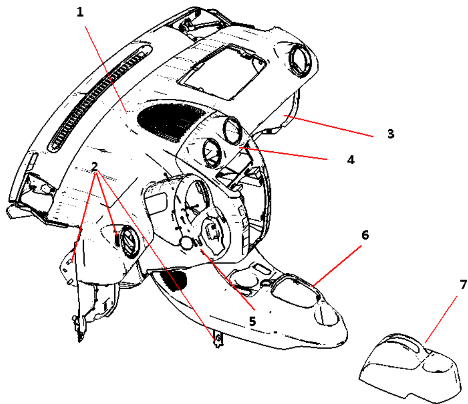
图 5.2.11 仪表台总成
