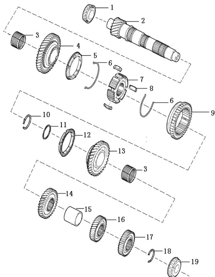
图 1.3.8 副轴组件
