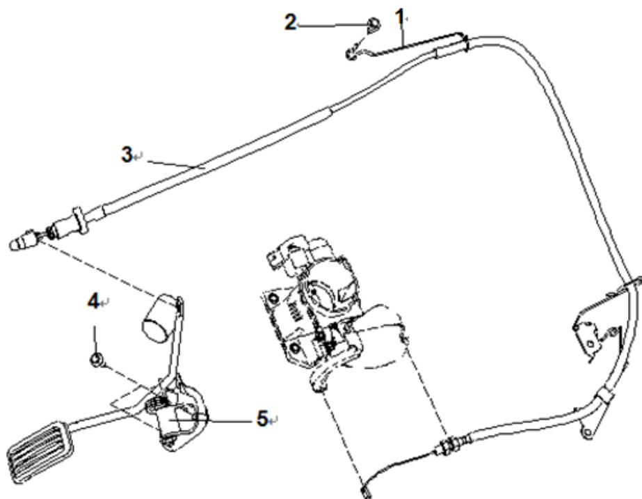
图 2.6.5 油门操纵机构总成
