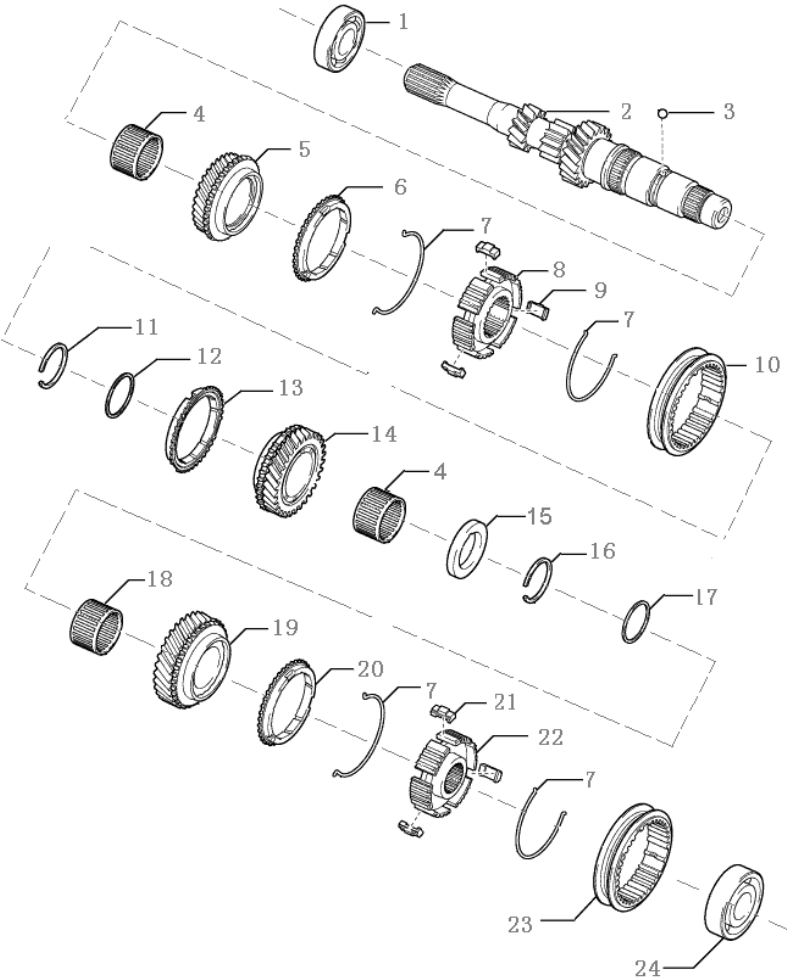
图 1. 2. 4 主轴组件
