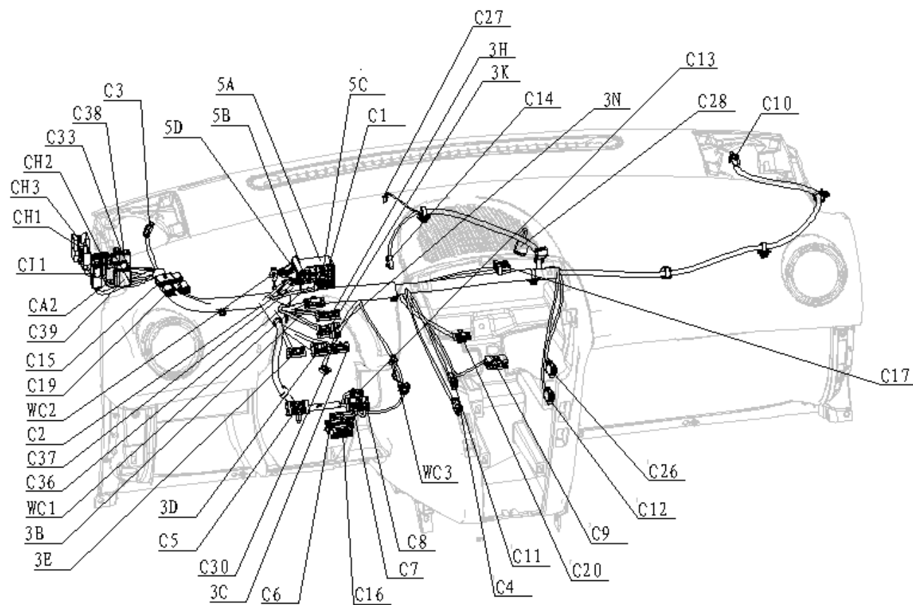
图 3.2.9 仪表线束
