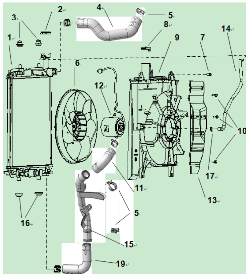
图 2.5.2 AMT 冷却系统
