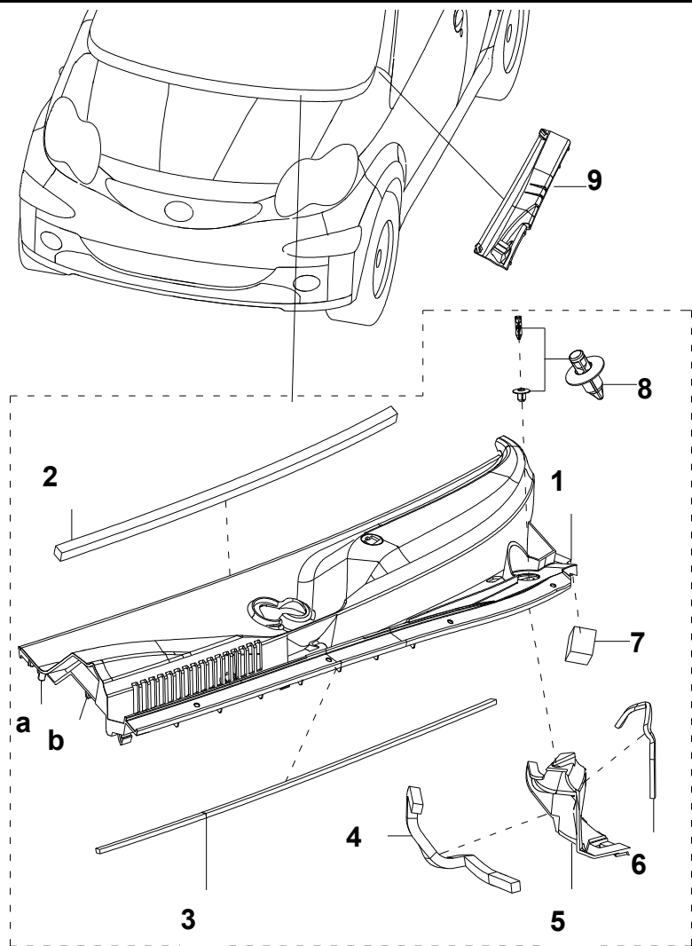
图 5. 1. 4 通风盖板右盖板及附件
