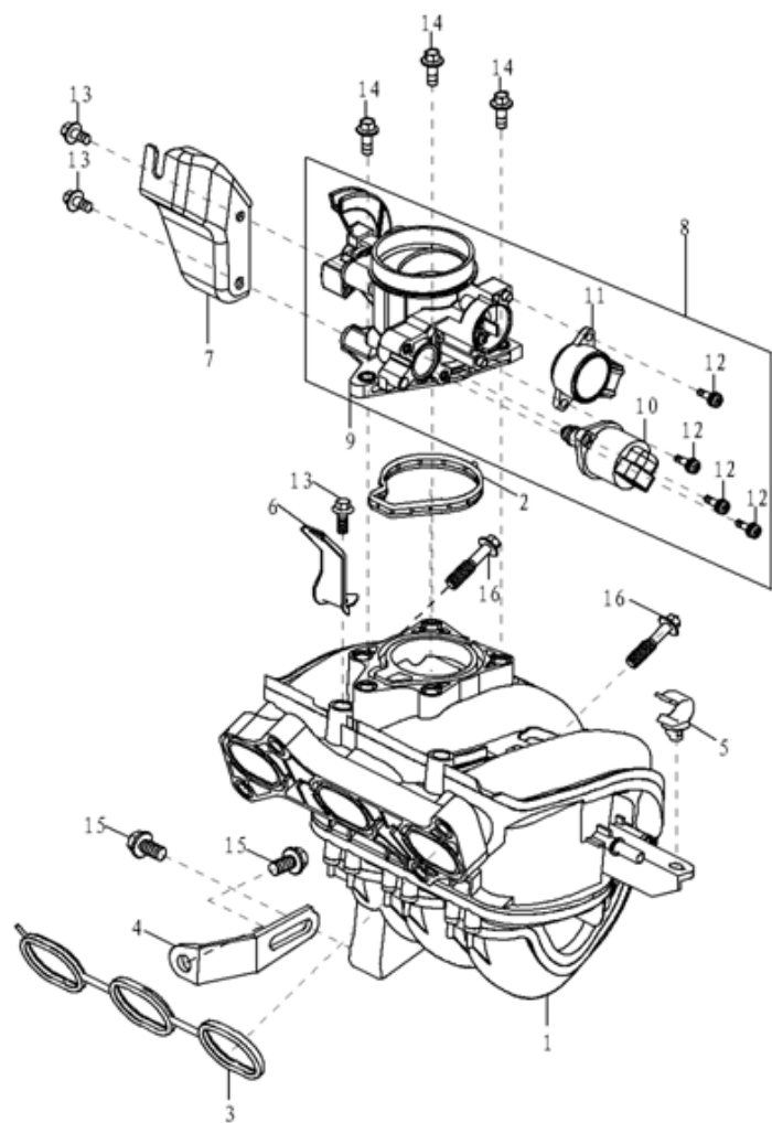
图 1. 1. 5 进气系统 (AMT)
