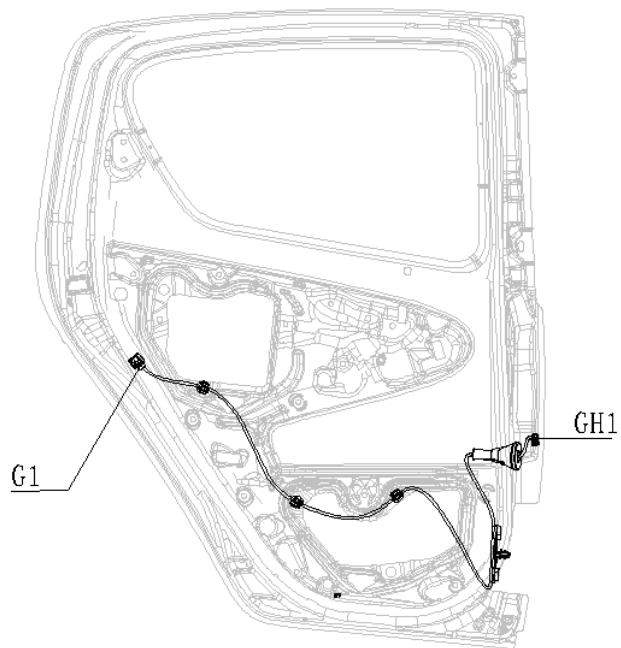
图 3.2.4 后门线束
