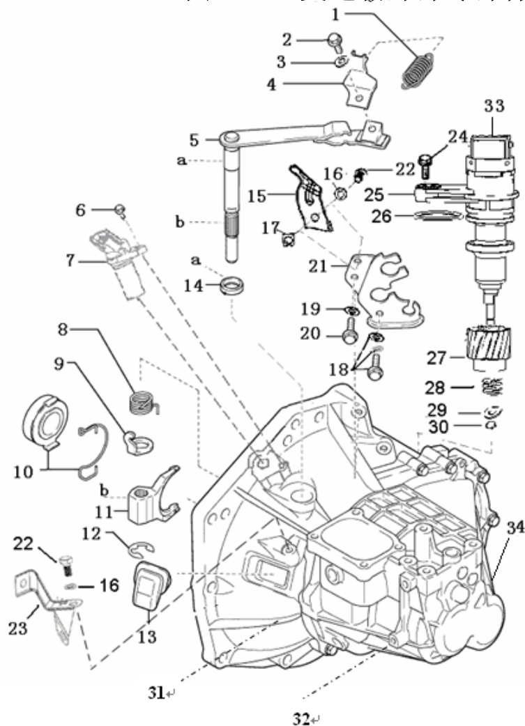
图 1.2.1 变速箱外部零部件
