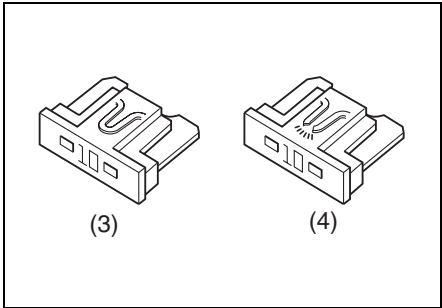
(3) 正常なヒューズの例 (4) 切れたヒューズの例
