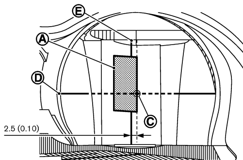
右側ヘッドランプ (単位: mm/インチ)
