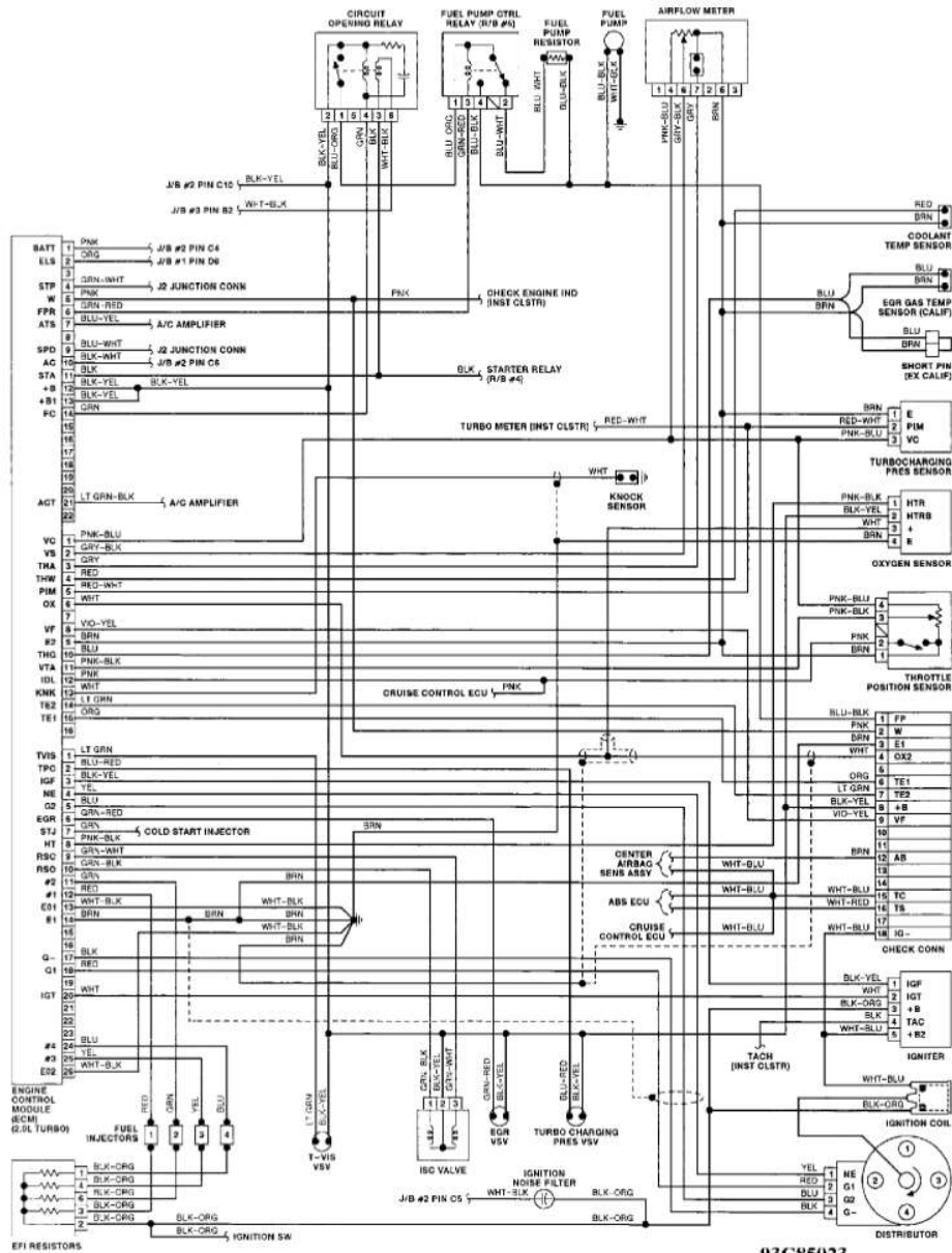
Fig. 2: Wiring Diagram (Celica 2.0L Turbo)
