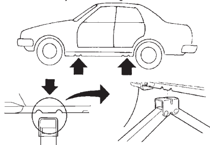
Punto de elevación y colocación del gato
