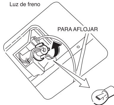
Luz de freno
