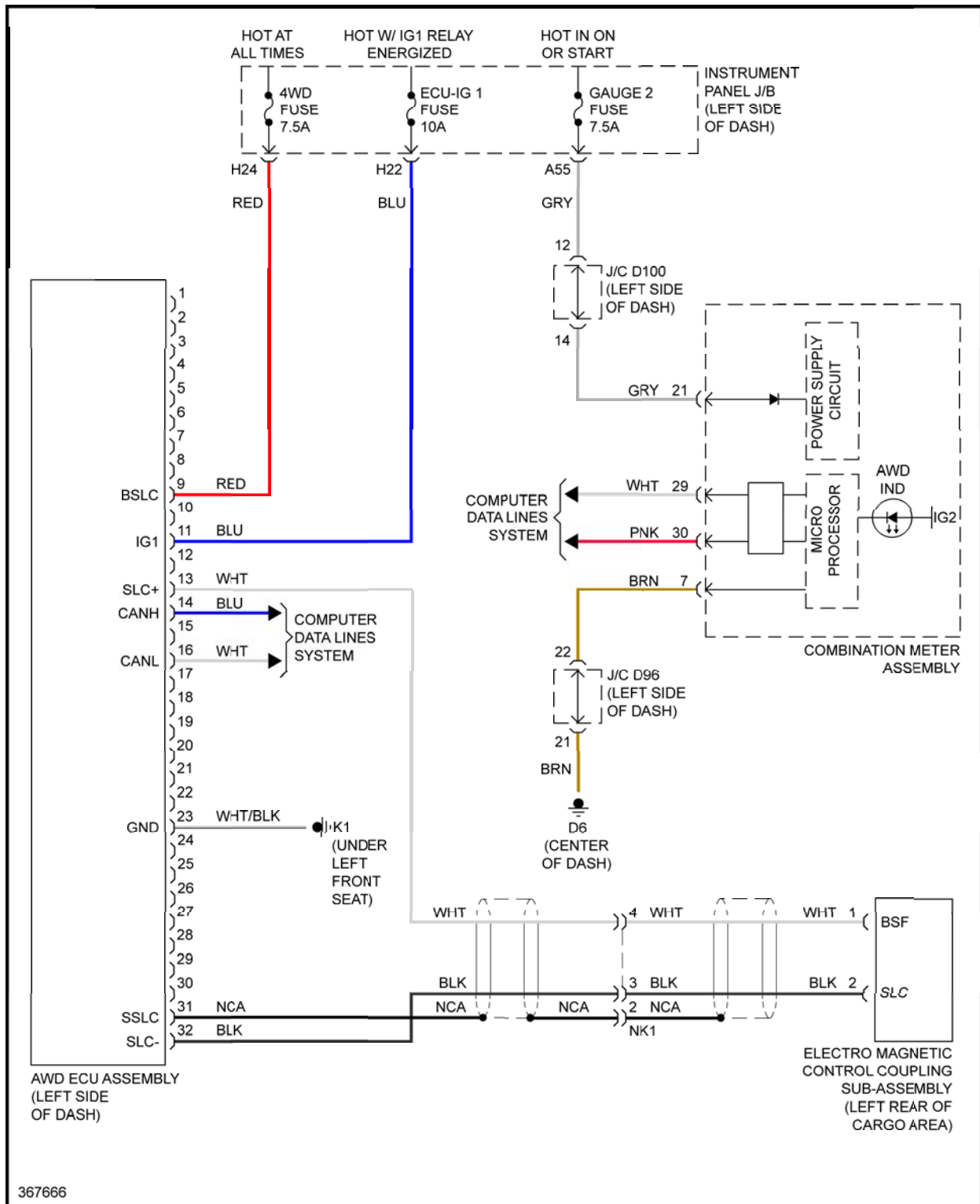
Fig. 113: 2.7L, AWD Circuit
